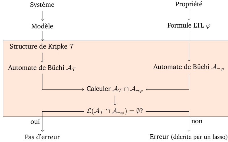
FIGURE 4.2 – Sommaire de l'approche de vérification algorithmique.
