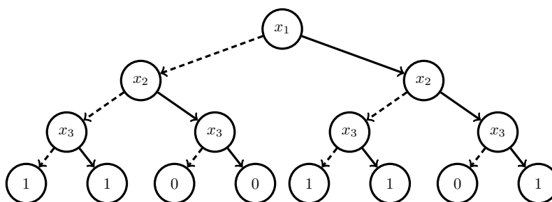
FIGURE 7.1 – Arbre de décision de l'expression booléenne (x_1 \vee \neg x_2) \wedge (\neg x_2 \vee x_3) . Une arête tillée (resp. pleine) sortant d'un sommet x_i indique la décision où la variable x_i prend la valeur faux (resp. vrai ). Les sommets 0 et 1 correspondent respectivement aux valeurs booléennes faux et vrai .
