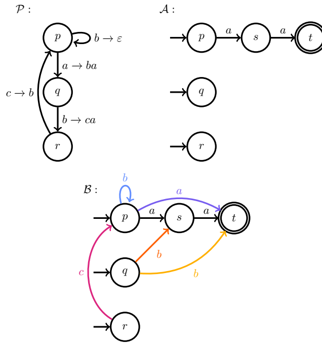
FIGURE 8.1 – Exemple de \mathcal{P} -automate \mathcal{B} tel que \text{Conf}(\mathcal{B}) = \text{Pre}^*(\mathcal{A}) calculé à partir d'un système à pile \mathcal{P} et d'un \mathcal{P} -automate \mathcal{A} .
