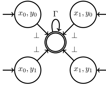
FIGURE 8.3 – Un \mathcal{P} -automate \mathcal{A} qui représente les configurations de \mathcal{P} où l'assertion est enfreinte, c.-à-d. \{ \langle (x_i, y_j), \perp w \rangle : i, j \in \{0, 1\}, w \in \Gamma^* \} .
